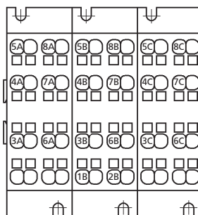
PRIR240 Modèle avec numérotation "TRIPOK" Vue arrière
