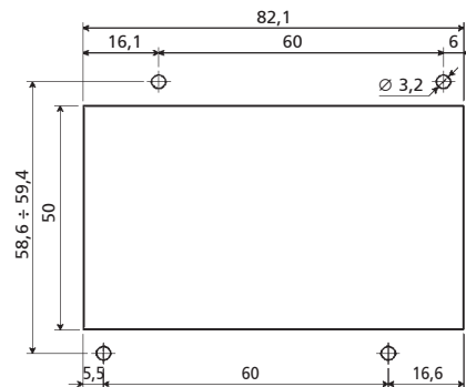
Gabarit de perçage
