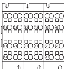
PRIR241 Modèle avec numérotation pour RVLV16/1
