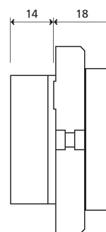
Vue latérale
