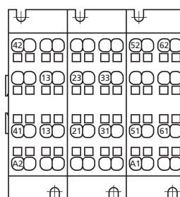
PRIR243 Modèle avec numérotation pour RVLV16/3
