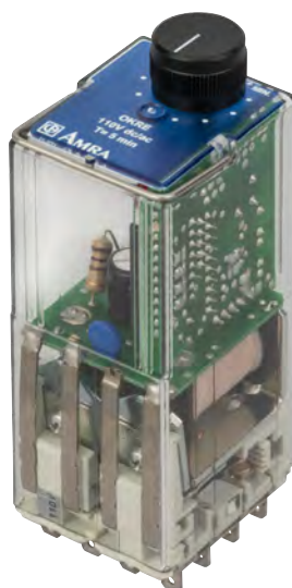
Temporisation réglage par bouton
