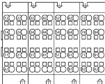
PRIR320 Vue arrière
