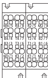
Vue arrière PRIR160
