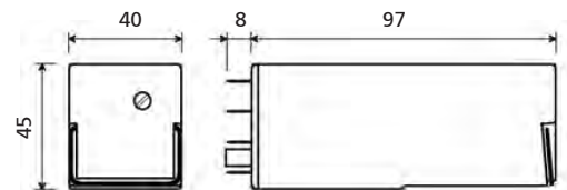
OKRE-L / OKRE-FP avec réglage par vis fendue à tête plate
