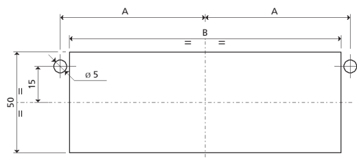
Gabarit de perçage
