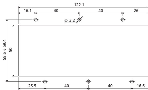
Gabarit de perçage
