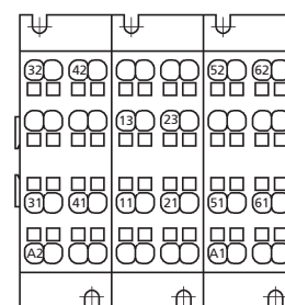
PRIR244 Modèle avec numérotation pour RVLV16/5
