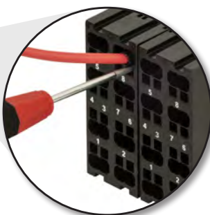
Détail des connexions
