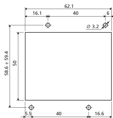
Gabarit de perçage
