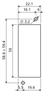
Gabarit de perçage
