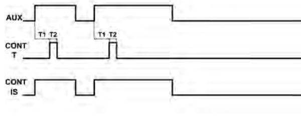
F7 – Fonction passage avec impulsion fixe (3 s), retardée à l'appel.
