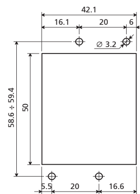
Gabarit de perçage
