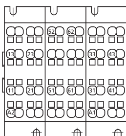
PRIR242 Modèle avec numérotation pour RVLV16/2
