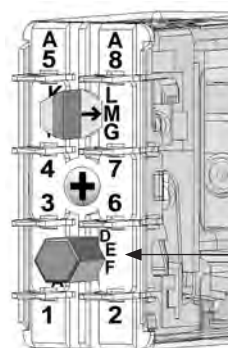
Exemple de sélection, pos. M sur relais POK
