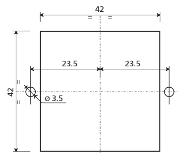
Gabarit de perçage
