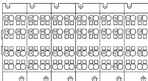
PRIR480 / Modèle avec numérotation "ESAPOK"
