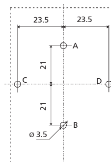
Gabarit de perçage
