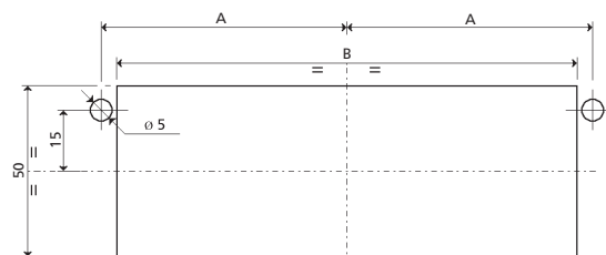
Gabarit de perçage
