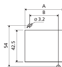
Gabarit de perçage
