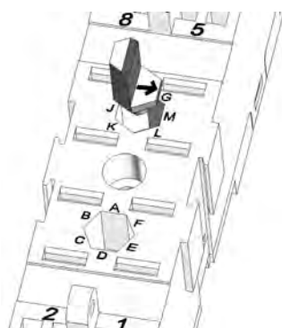
Exemple de sélection, pos. M sur embase à 8 encoches
