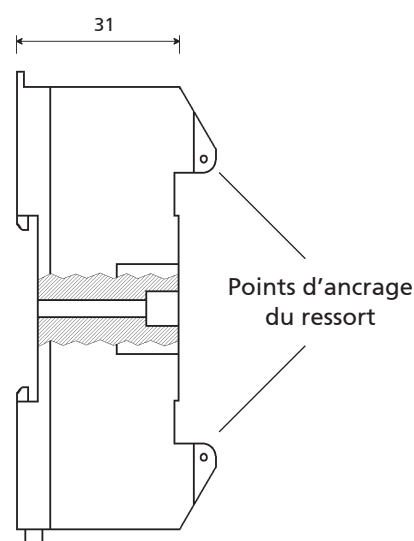
Vue latérale
