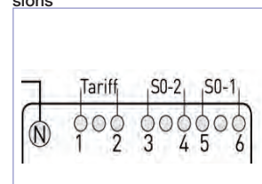
Entrées tarif &amp; sorties impulsions
