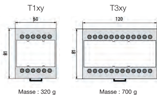
Masse : 320 g
