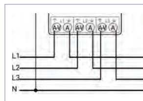
4 fils, 3 courants
